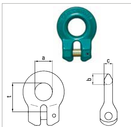
Gabelverbinder Eye-Connector
